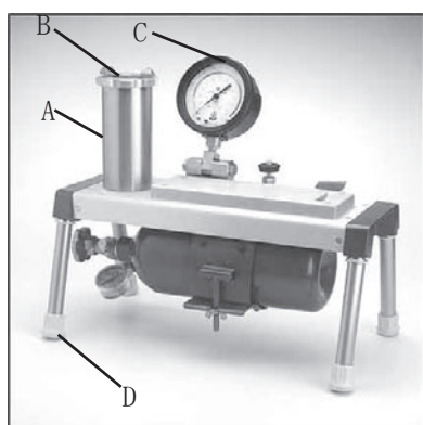
3005, 植物水分状態制御装置
