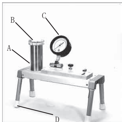
3000, 植物水分状態制御装置
